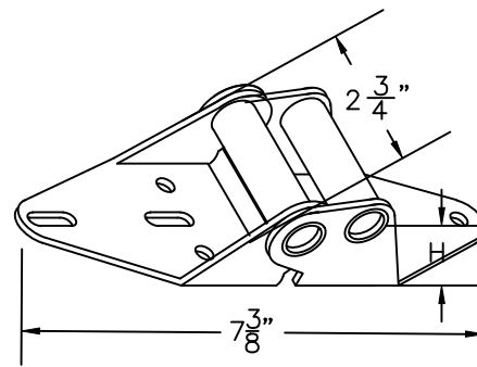
END HINGE
